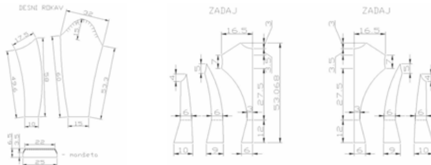
Kroj »kočemajke« izrisal Filip Pakiž v programu AutoCAD.
